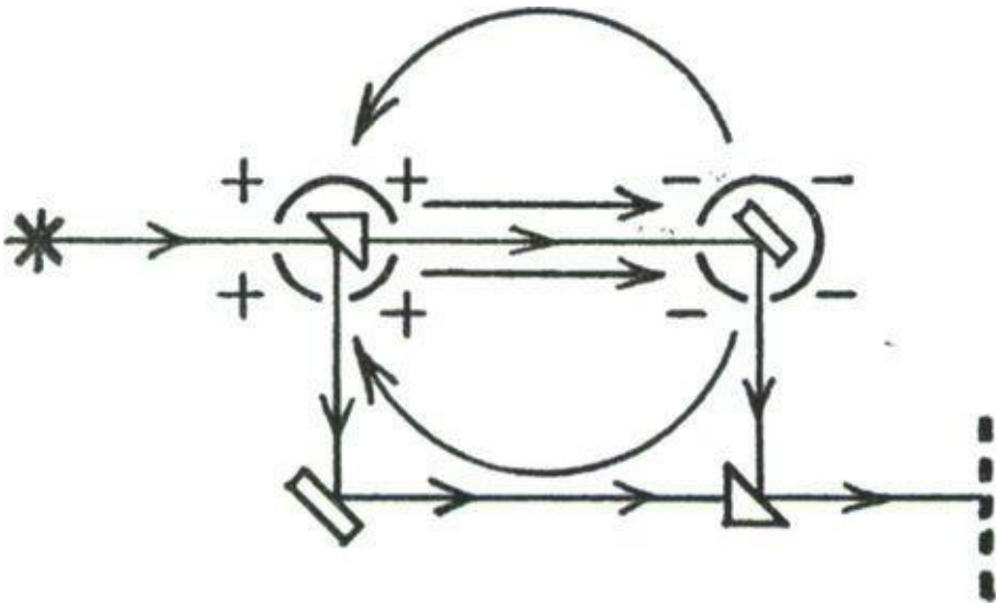
Krafft’s Interferometer
